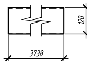
поз.17 (М1:10) Гн. 120x4x3738 С245
