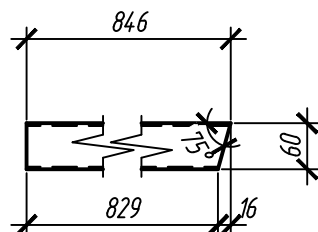
поз.10 (М1:10) Гн. 60x3x846 С245
