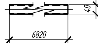
поз.25 (М1:10) Гн. 40x3x6820 С245
