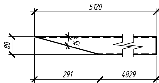
поз.14 (М1:10) Гн. 80x3.5x5120 С245
