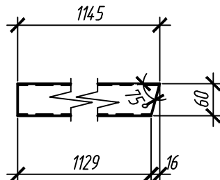
поз.9 (М1:10) Гн. 60x3x1145 С245
