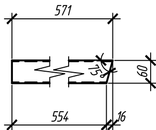
поз.3 (М1:10) Гн. 60x3x571 С245
