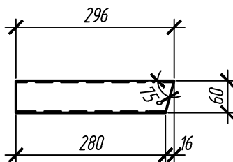
поз.5 (М1:10) Гн. 60x3x296 С245
