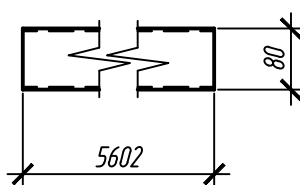
поз.13 (М1:10) Гн. 80x3.5x5602 С245
