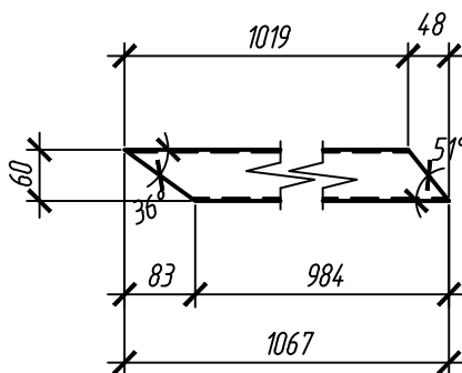
поз.5 (М1:10) Гн. 60x3x296 С245
